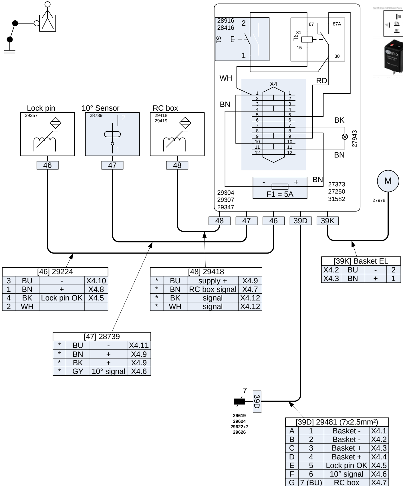
Diagram for E kurv på Flyjib. Tidsbegrænset signal for pinlock ved af og på montering
